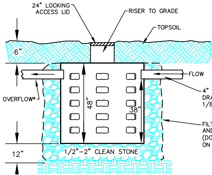
ELEVATION
